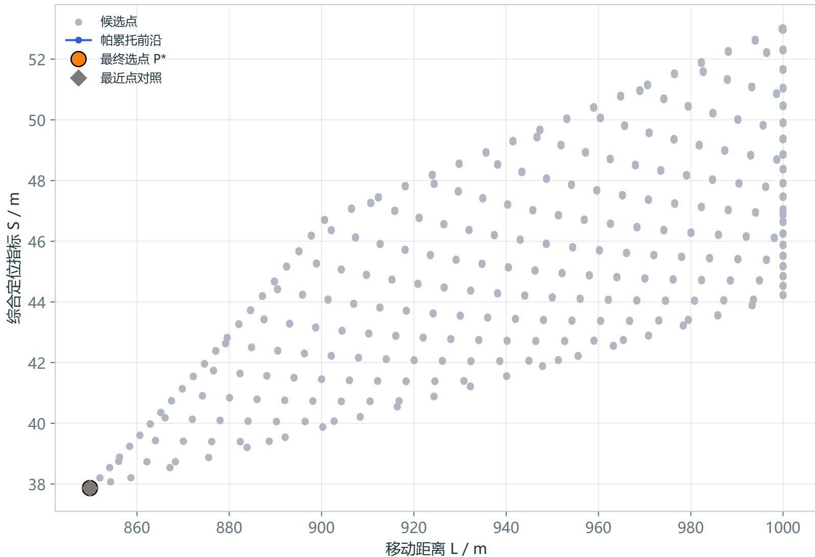
距离与定位指标的帕累托关系 ( \Delta L=0.0 m, \Delta S=0.0 m, \lambda_0=0 )
